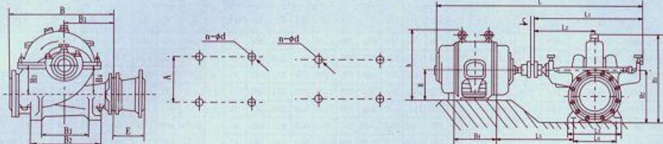
外形安装尺寸表(不带底座)
